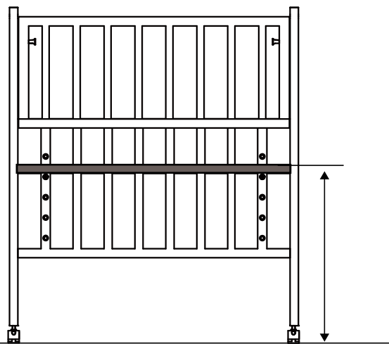
床板高さH=54cm
