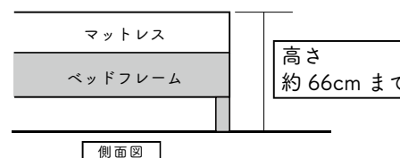
側面図
